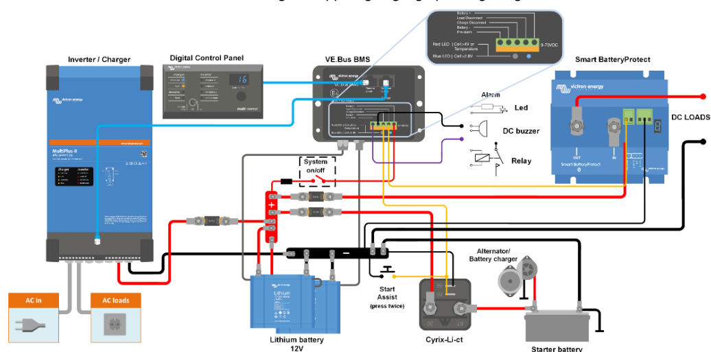
Abbeelding 1: Toepassingsvoorbeeld voor een voertuig of boot.
