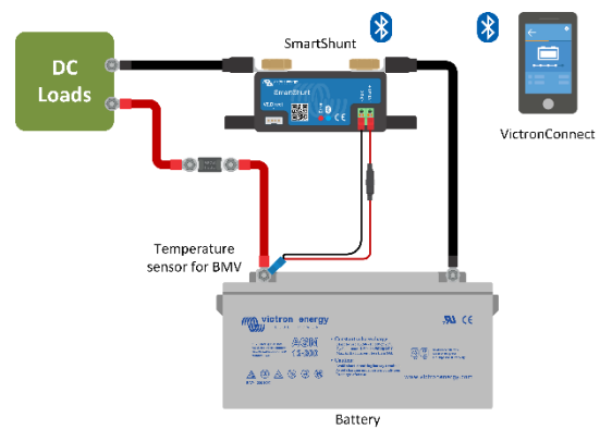
Metten batterijtemperatuur
