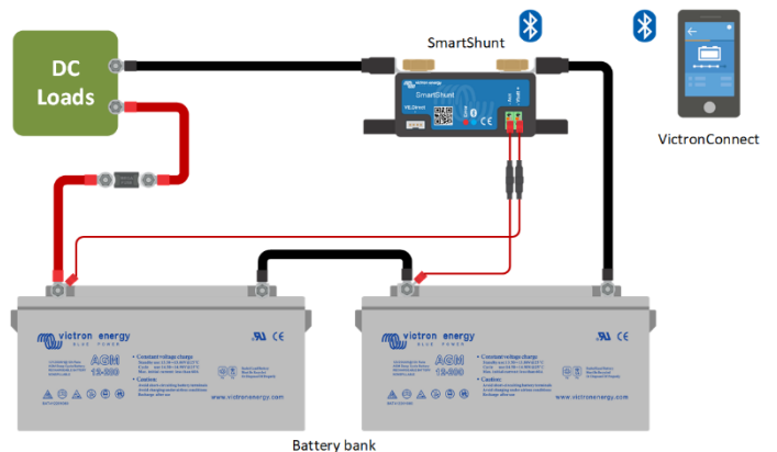
Metten middelpunt batterijbank
